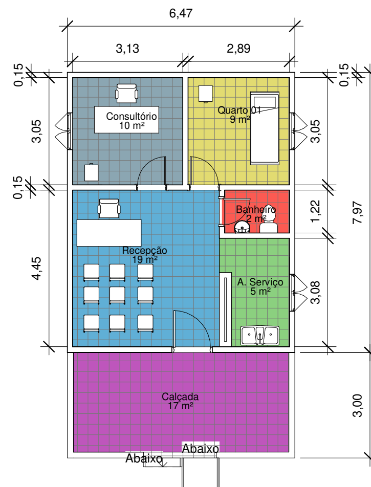
1 Planta Baixa do Pav. Térreo 1 : 100
