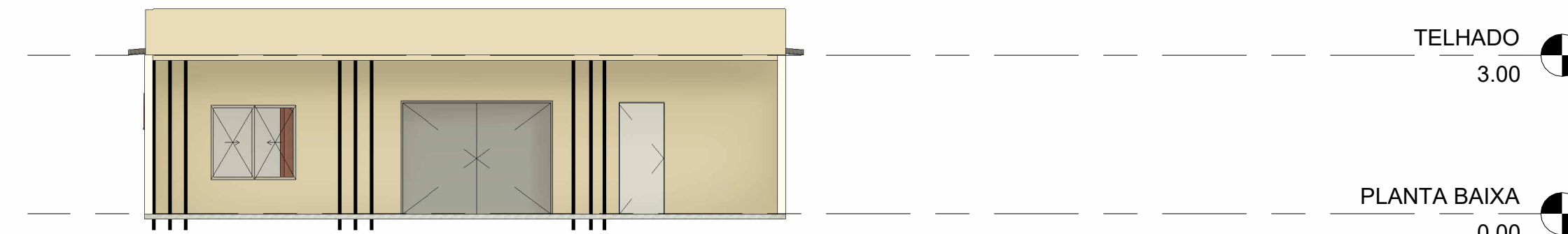
4 VISTA FRONTAL 1 : 100
