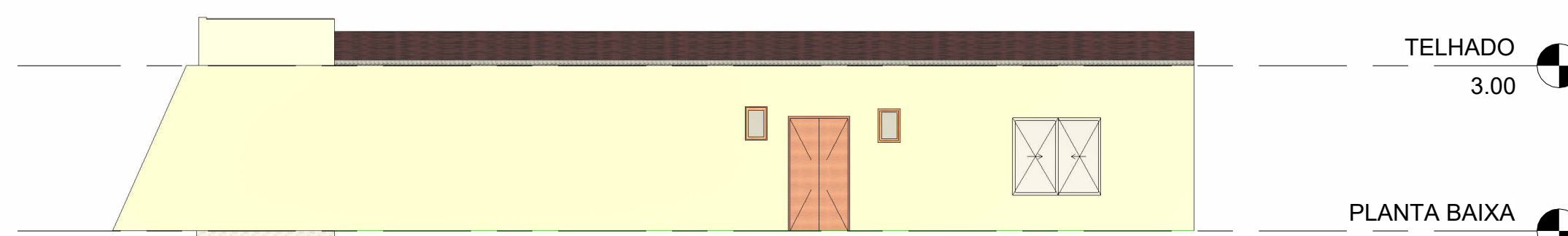
2 VISTA LATERAL 1 : 100
