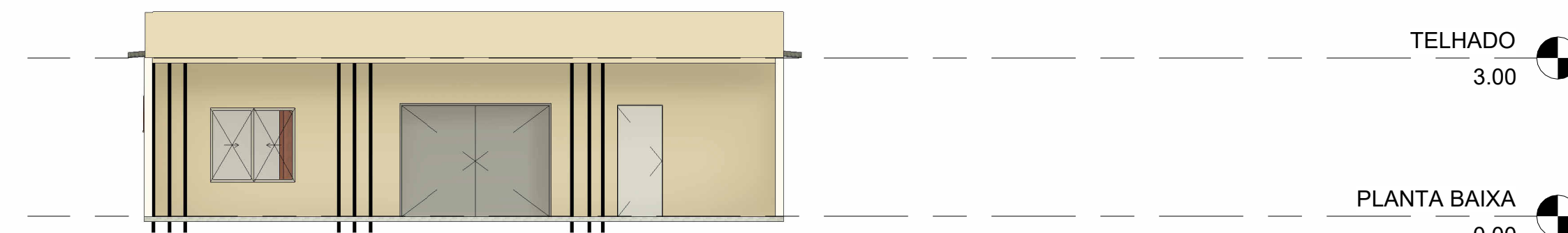
4 VISTA FRONTAL 1 : 100
