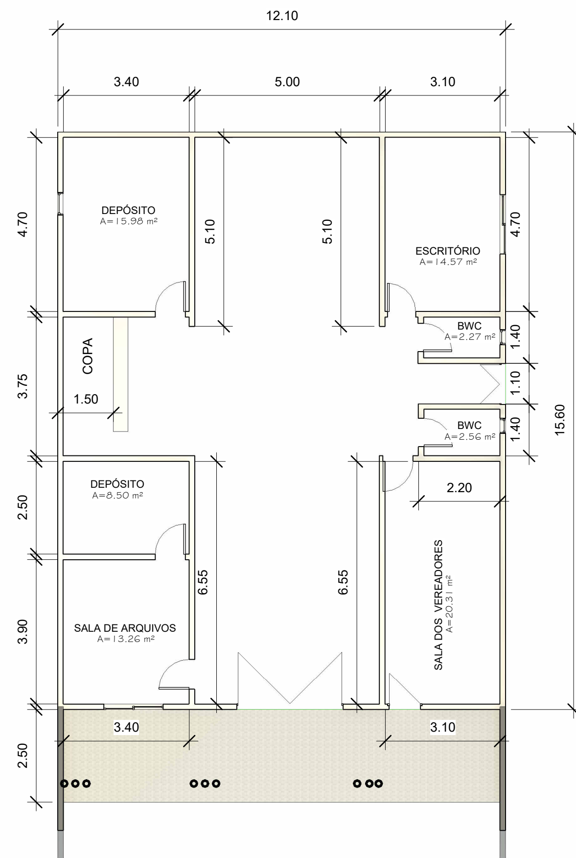
1 PLANTA BAIXA 1 : 100
