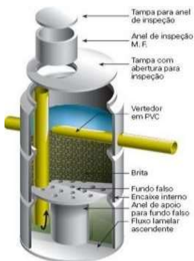
Figura 7 – Exemplos de tanques anaeróbios. Fonte: http://www.ecoeficientes.com.br/ (2014).
