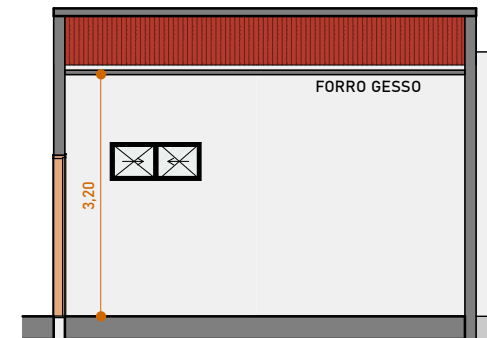
3 | Corte 1 1 : 100
