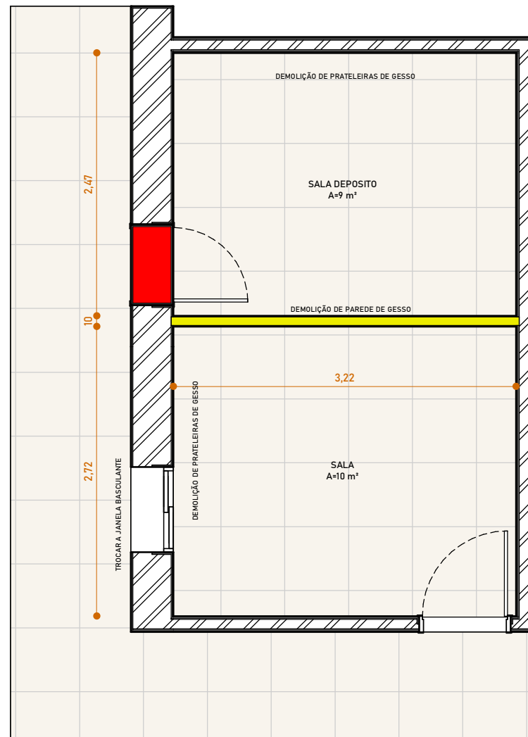
1 | TÉRREO - EXISTENTE 1 : 50
