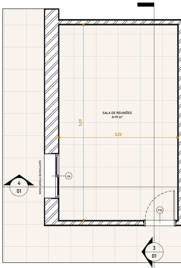
2 | TÉRREO - NOVO LAYOUT 1 : 50
