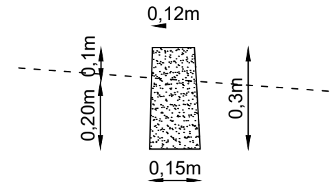
MEIO-FIO DE CONCRETO PRÉ-MOLDADO
