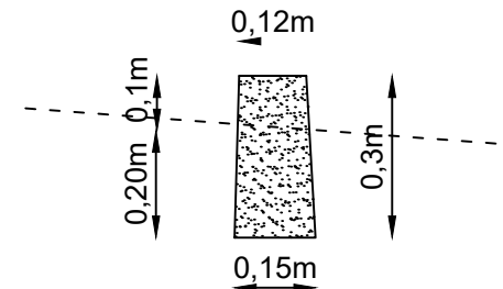
MEIO-FIO DE CONCRETO PRÉ-MOLDADO
