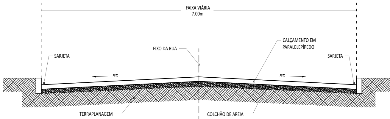
TRANSVERSAL ESC. 1:50
