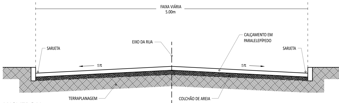
TRANSVERSAL ESC. 1:50
