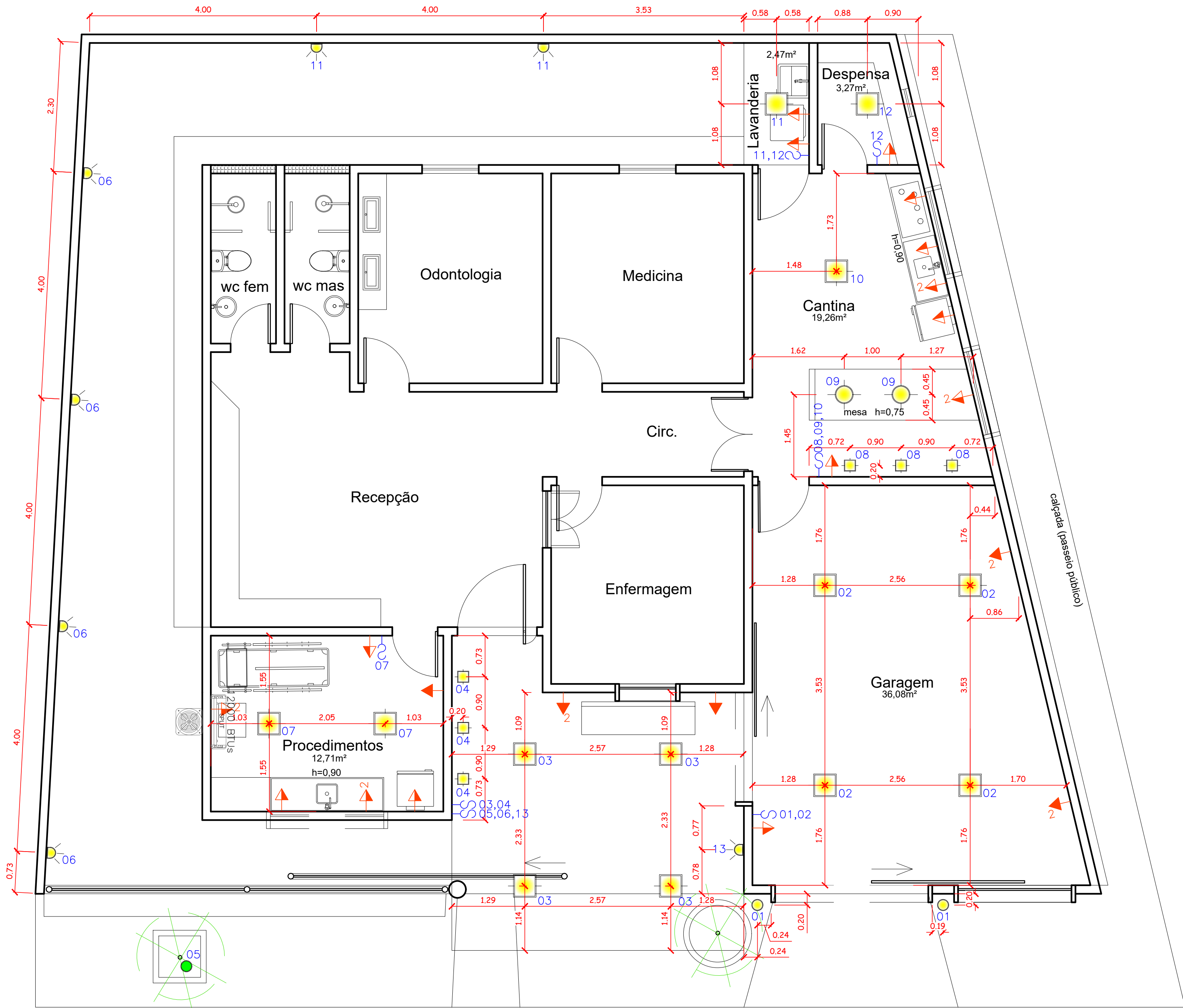
PLANTA LUMINOTÉCNICA ESCALA 1/50
